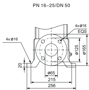
FLANGE DIN(LVR)/F
