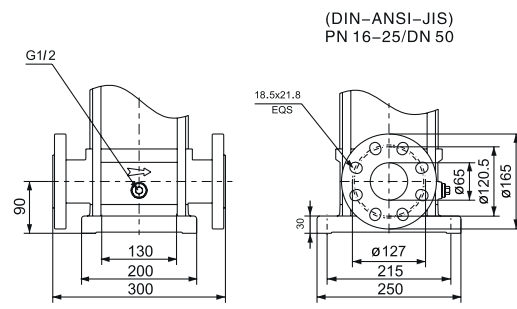
FLANGE DIN(LVS)/F
