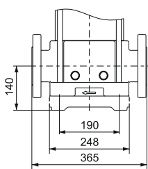
FLANGE DIN(LVR)/F
