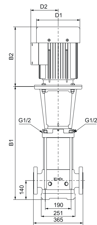
FLANGE DIN(LVS)/F
