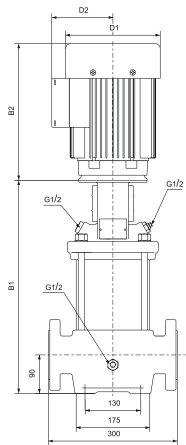
FLANGE DIN(LVR)/F
